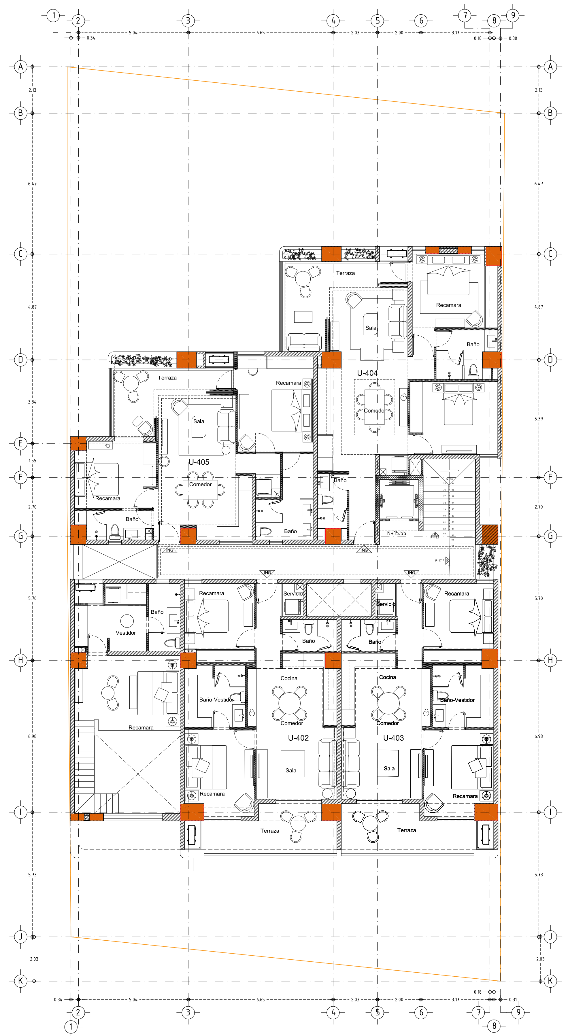
NIVEL 4
