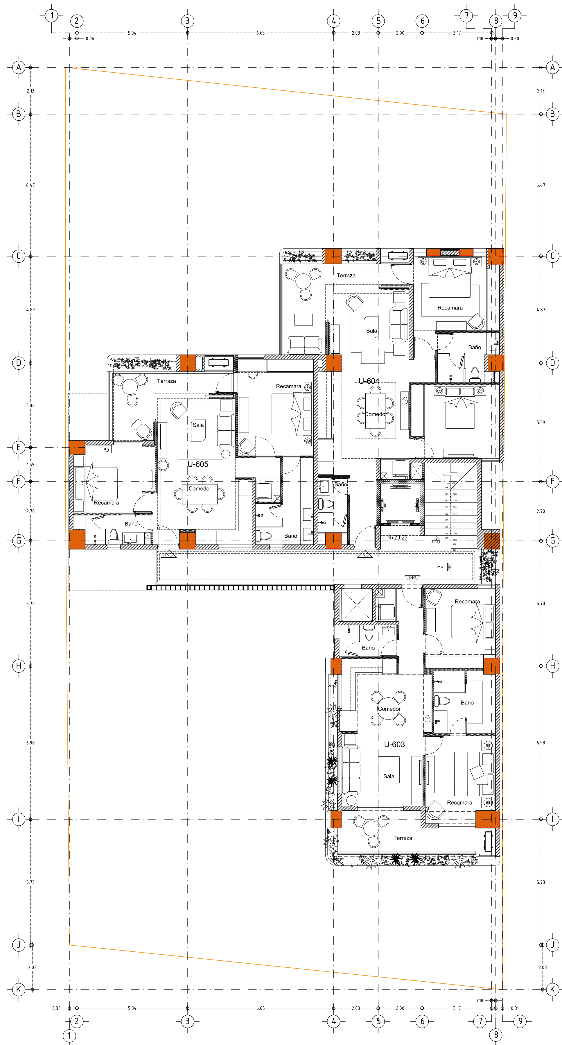
NIVEL 6
