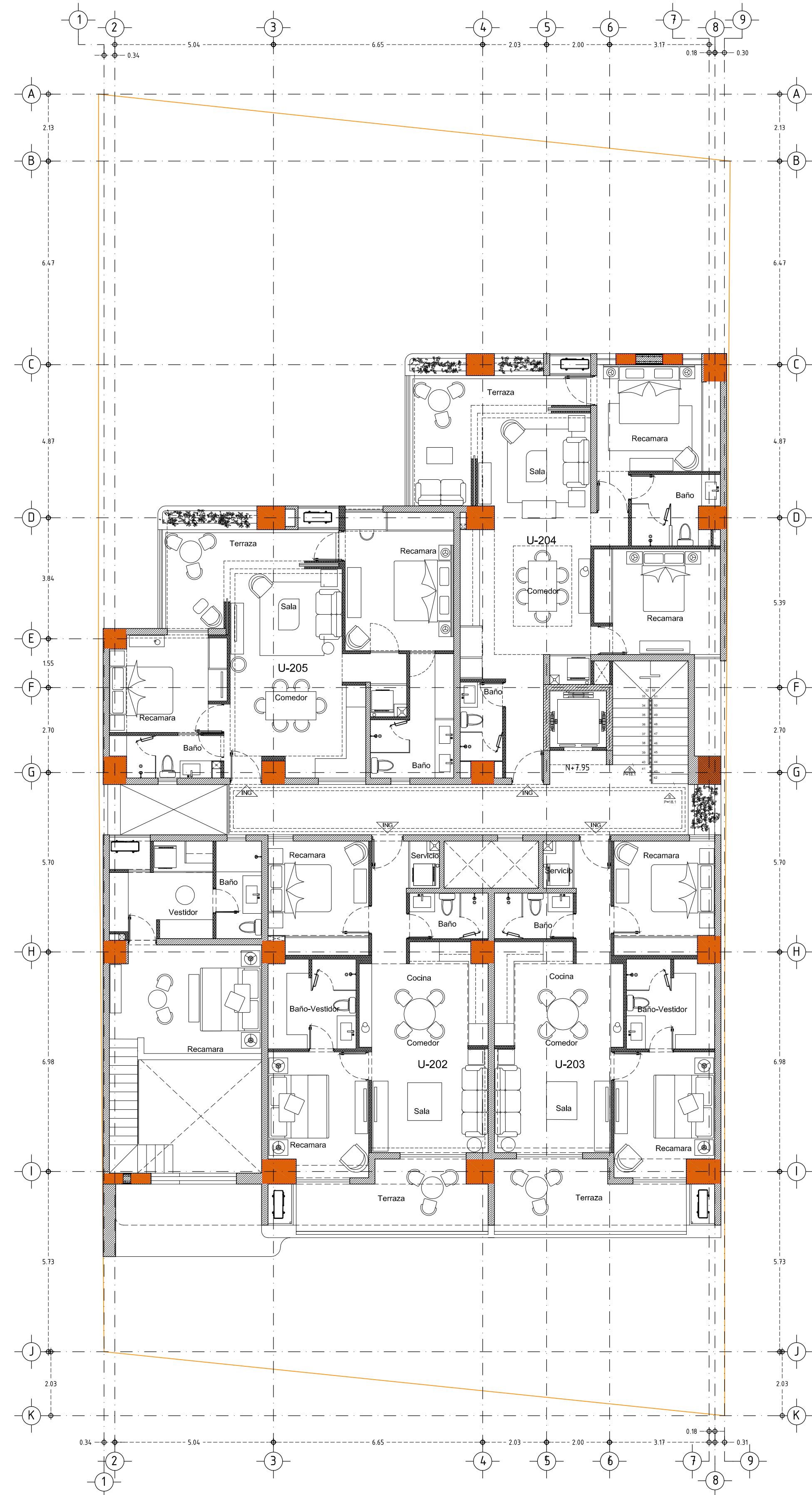
NIVEL 2
