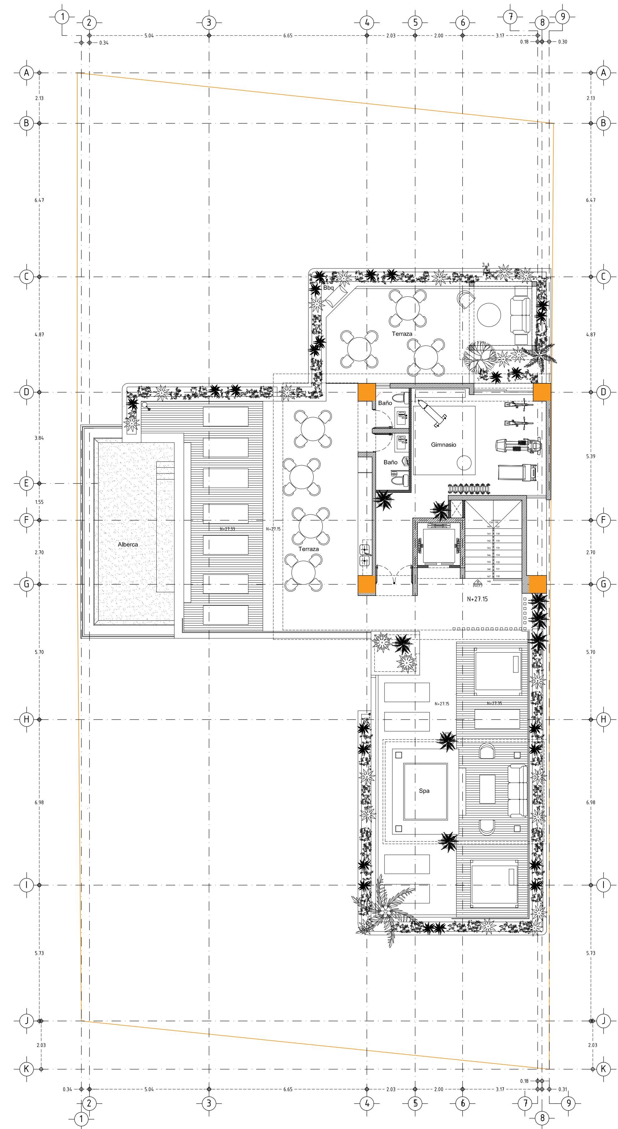
NIVEL 7
