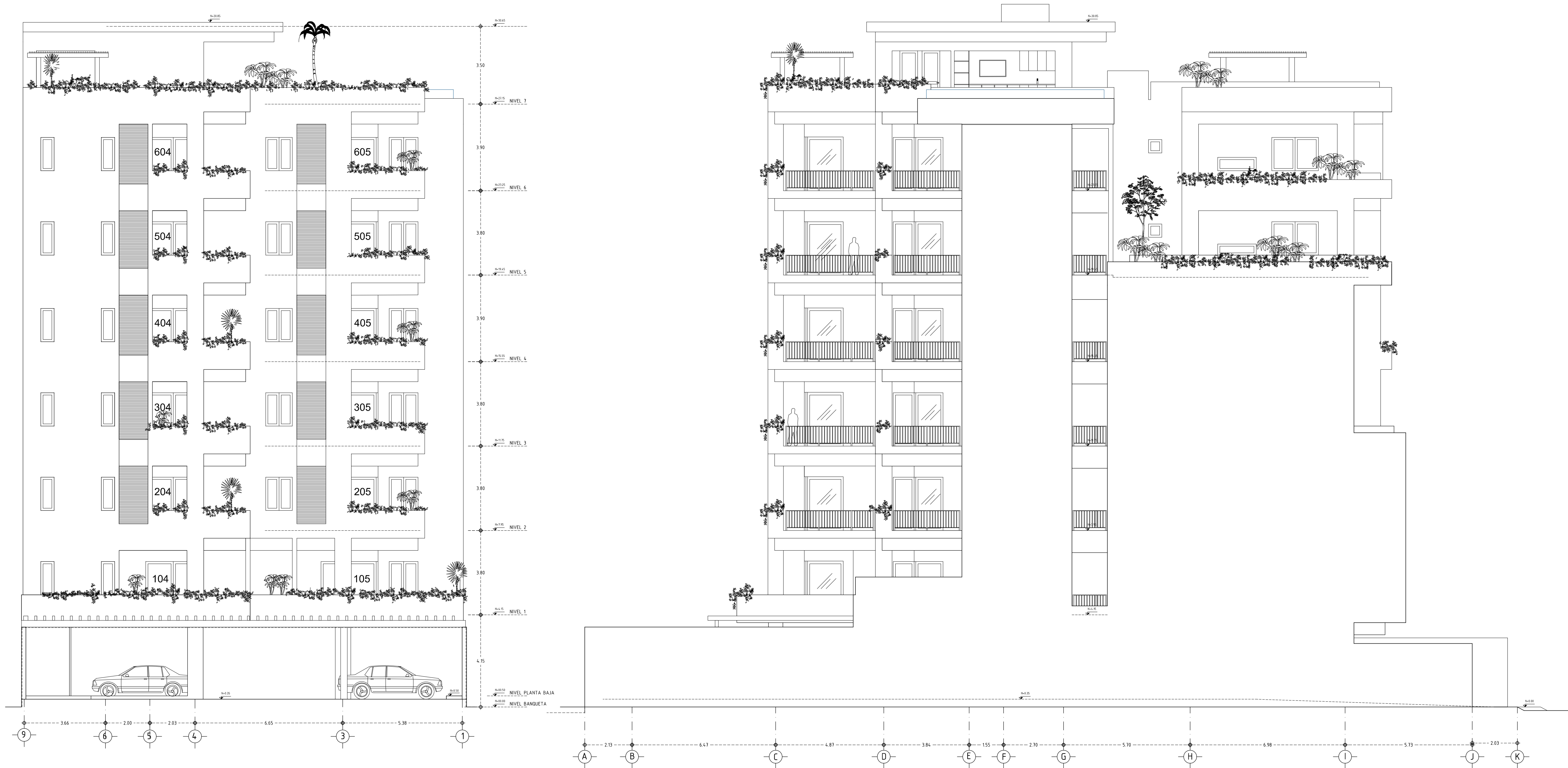
ALZADO POSTERIOR
