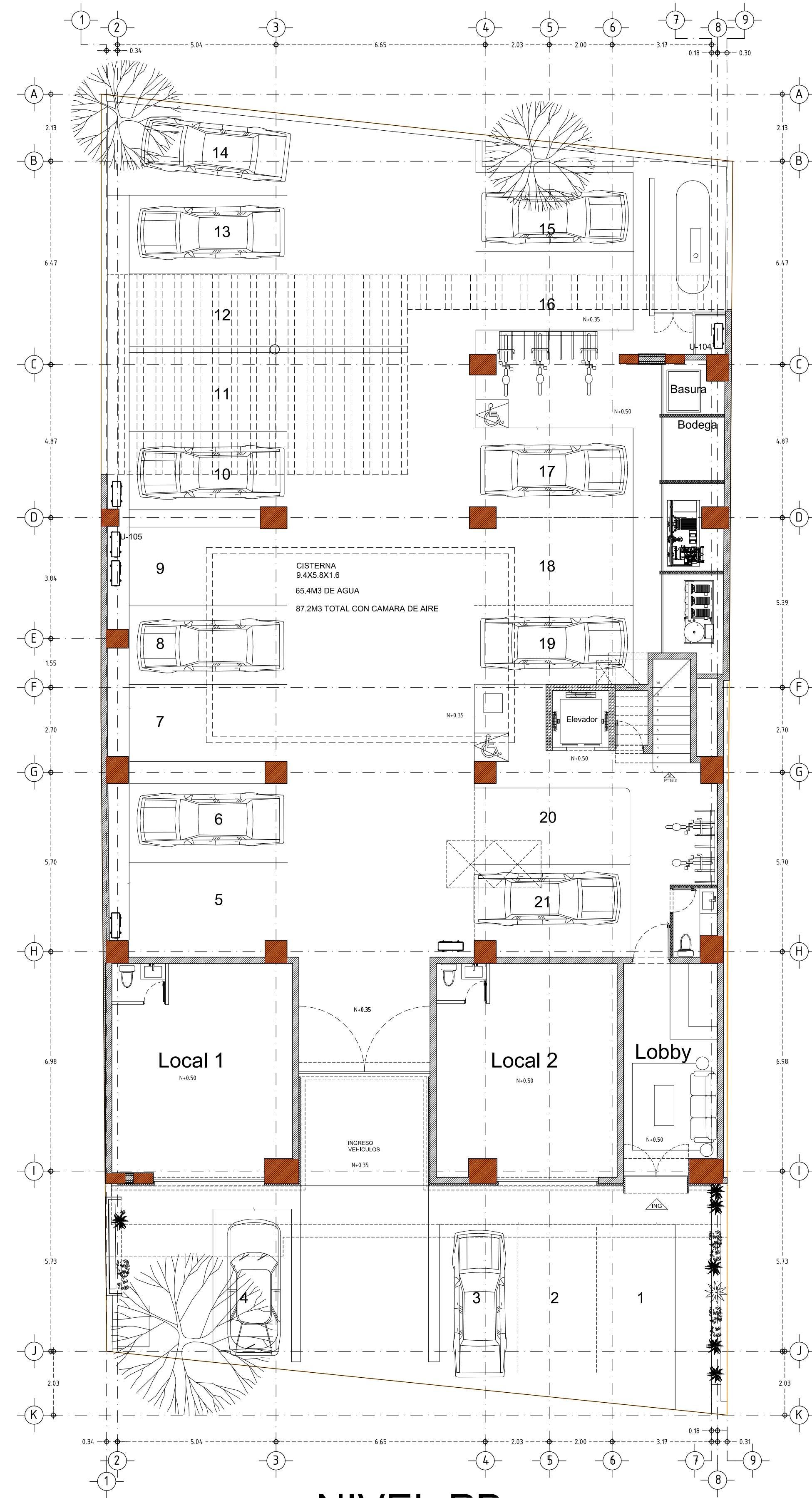
NIVEL PB
