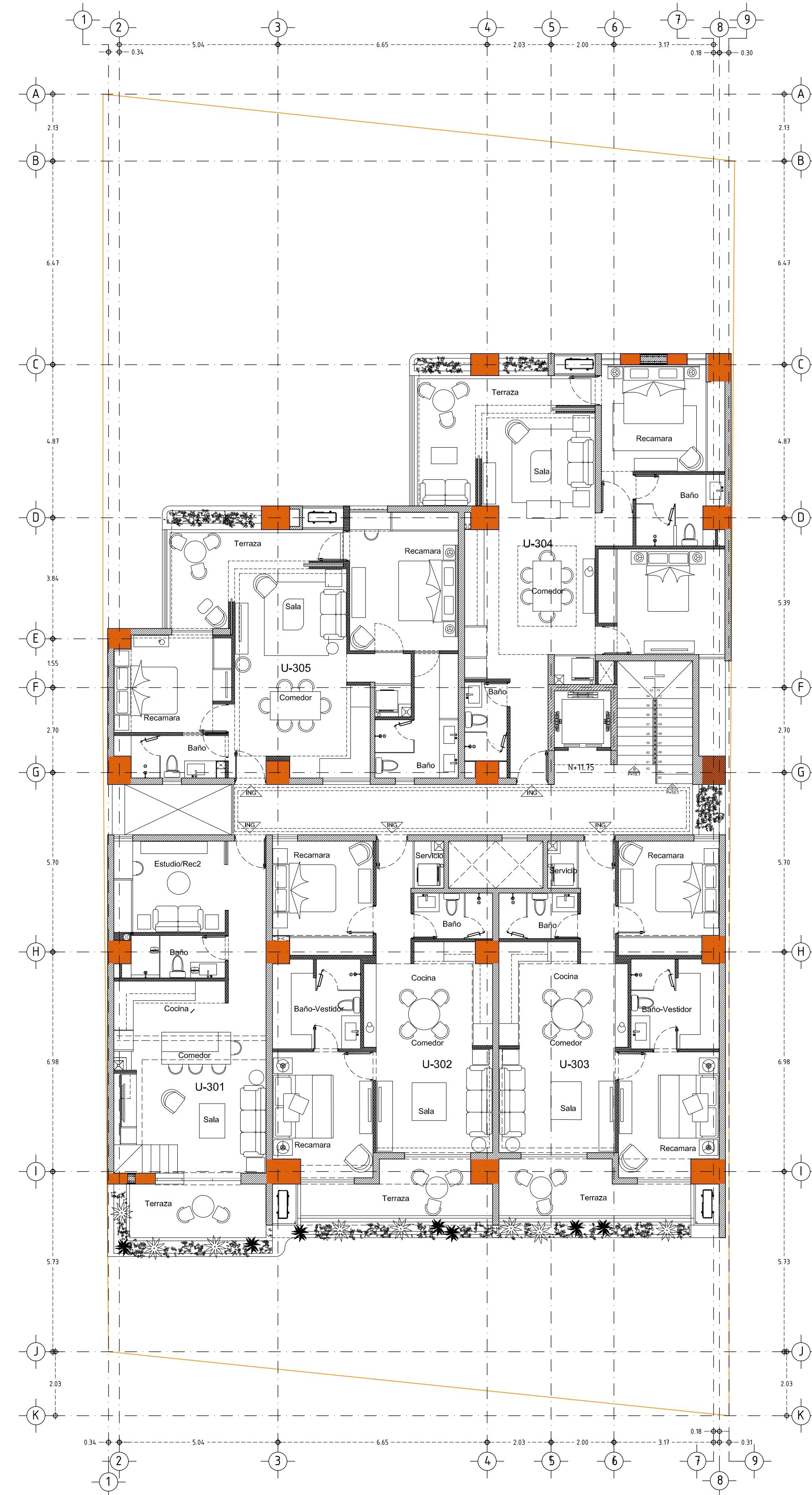
NIVEL 3
